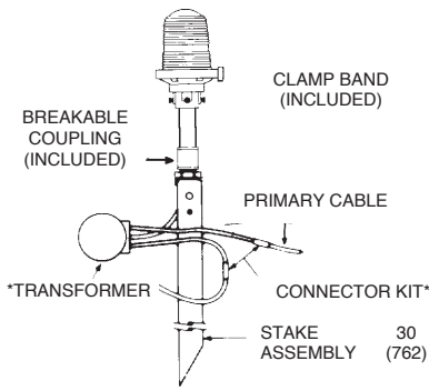
Stake Mounted ERL
