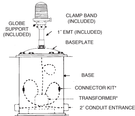
Base Mounted ERL
